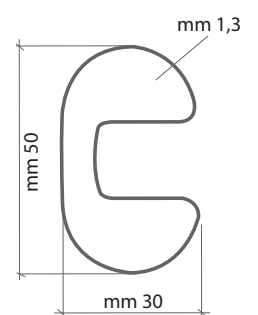
Sezione telaio
