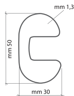
Sezione telaio
