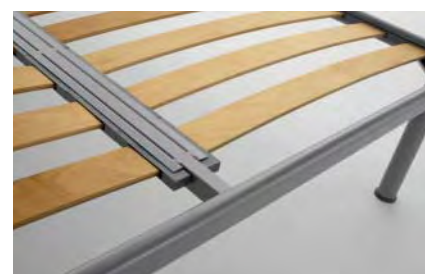
sistema incasso listelli su supporto centrale
