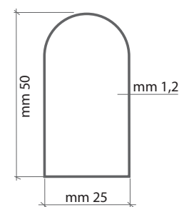
Sezione telaio
