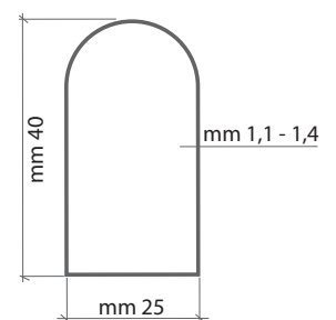
Sezione telaio
