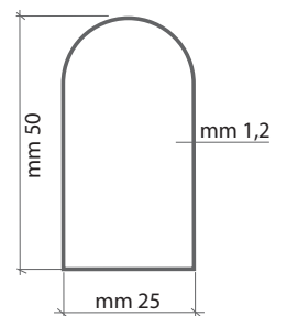
Sezione telaio
