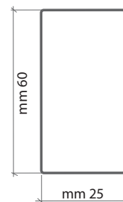
Sezione telaio
